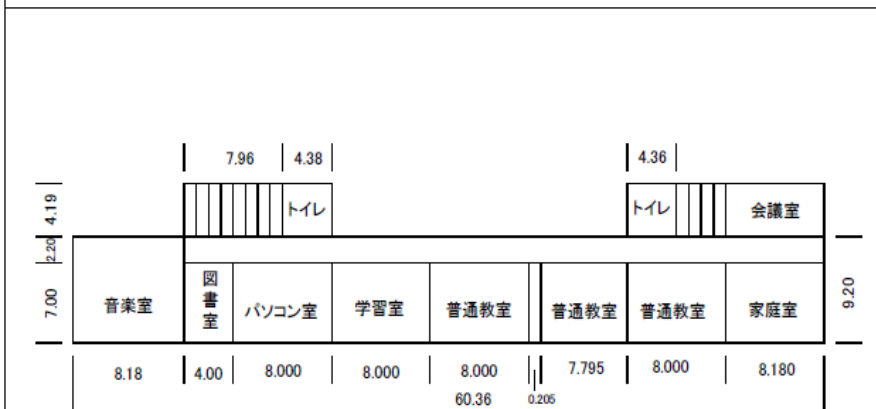
① 2階平面図
