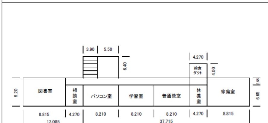
① 2階平面図
