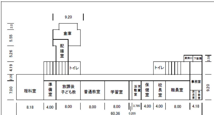
① 1階平面図
