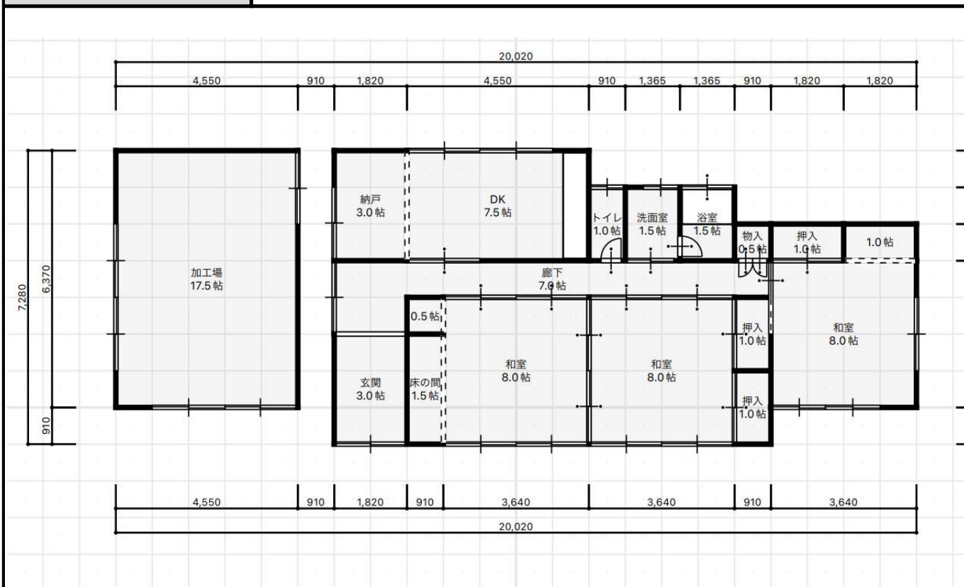
(11)配置図・間取り図
